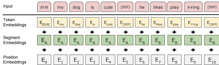
Gambar 2.8: Representasi input BERT yang terdiri dari token , segment , dan position embedding (Devlin et al. , 2018)
