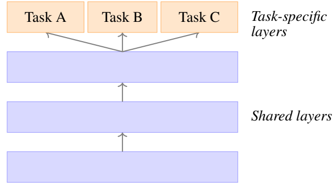
Gambar 2.12: Ilustrasi arsitektur hard parameter sharing dalam Multi-Task Learning (Ruder, 2017, telah diolah kembali)
