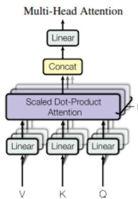
Gambar 2.11: Mekanisme Scaled Dot-Product Attention pada Multi-Head Attention (Vaswani et al., 2017)
