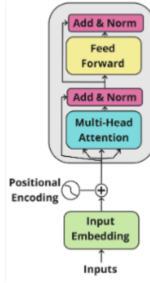
Gambar 2.10: Struktur satu lapisan Transformer Encoder (Devlin et al. , 2018)
