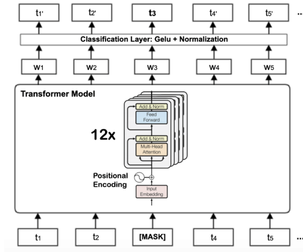
Gambar 2.9: Tumpukan L lapisan Transformer Encoder pada BERT (Devlin et al. , 2018)
