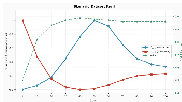
Gambar 4.3: Skenario dataset kecil: \mathcal{L}_{\text{sent}} mencapai kondisi stabil lebih dahulu, kemudian \mathcal{L}_{\text{clust}} mulai menurun dan kedua komponen menunjukkan pola yang lebih seimbang.
