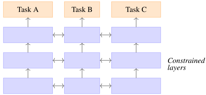
Gambar 2.13: Ilustrasi arsitektur soft parameter sharing (Ruder, 2017, telah diolah kembali)
